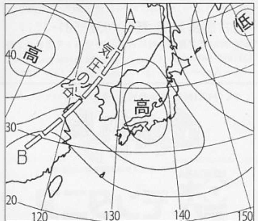
地上天気図にみられる気圧の谷
