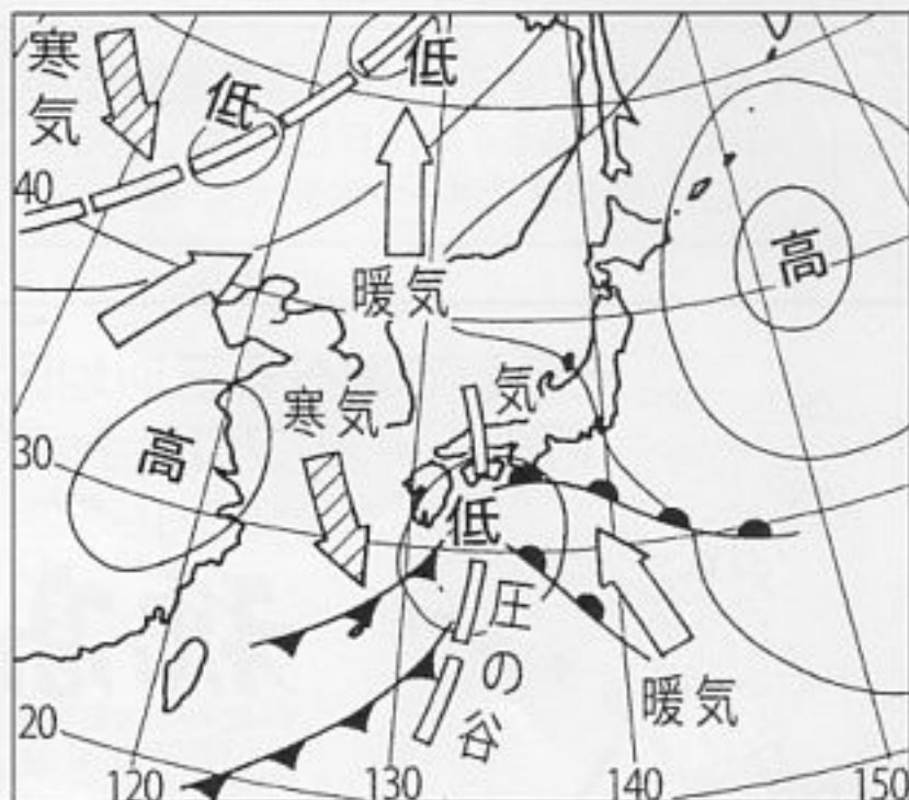
地上天気図にみられる気圧の谷
